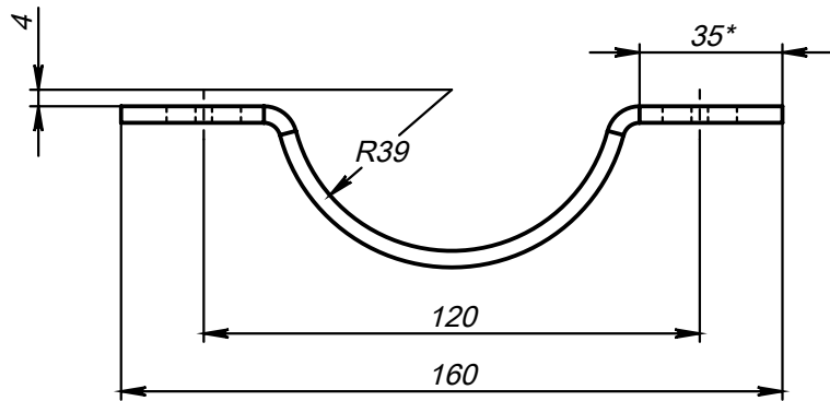
Поз.2 (Полухомут)
