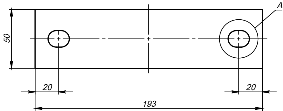
Поз.2 (Полухомут) развертка
